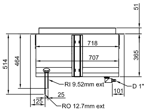
Zadní strana
